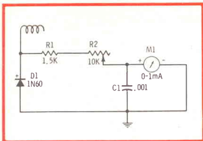
Fig. 8 - Piccolo misuratore di segnali per il controllo di emissione di un trasmettitore mobile.
