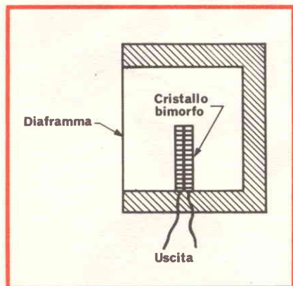
Fig. 10 - Schema costruttivo del microfono piezoelettrico o ceramico.
