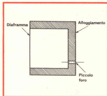
Fig. 1 - Microfono a pressione.
