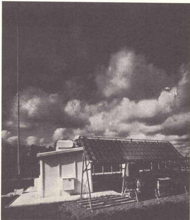
Fig. 38 - Batteria di celle solari al silicio BPX46/47 (Philips) per impieghi terrestri.
