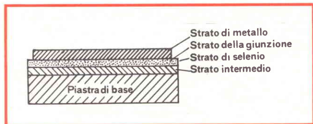
Fig. 40 - Struttura schematica di una fotocella al selenio.
