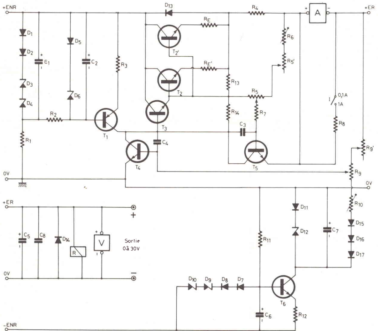
Fig. 18 - Schema completo della parte elettronica dell'alimentatore stabilizzato. In basso a sinistra è riprodotto il circuito attraverso il quale viene controllata l'entità della tensione disponibile in uscita.
