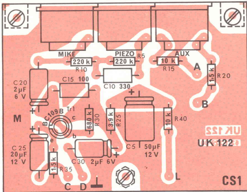
Fig. 2 - Disposizione dei componenti sulla basetta a circuito stampato C.S.1.
