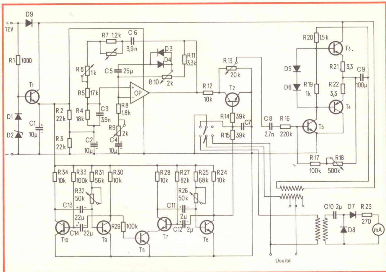
Fig. 5 - Progetto di circuito come trasmettitore di segnalazione di percorso.
