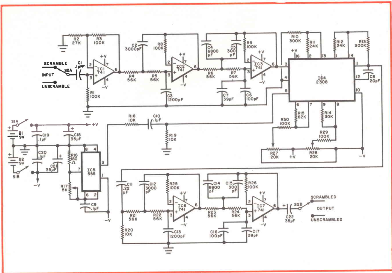
Fig. 5-B - Schema elettrico completo dell'intera apparecchiatura: il funzionamento si basa sul fatto che i valori di frequenza vengono tra loro invertiti, in modo da rendere il messaggio assolutamente inintelligibile, se non dopo aver riconvertito le diverse frequenze dei segnali che lo compongono, attraverso un'apparecchiatura identica alla prima, ma funzionante in senso opposto.
