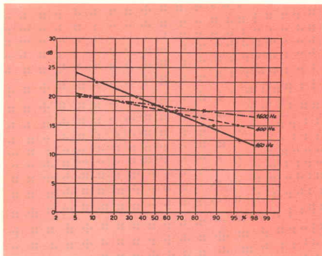
Fig. 6 - Distribuzione statistica dei livelli relativi di pressione sonora su carta gaussiana: la sorgente è un altoparlante posto nel punto 1 (v. fig. 3), alimentato con suono bianco filtrato per terzi di ottava.
