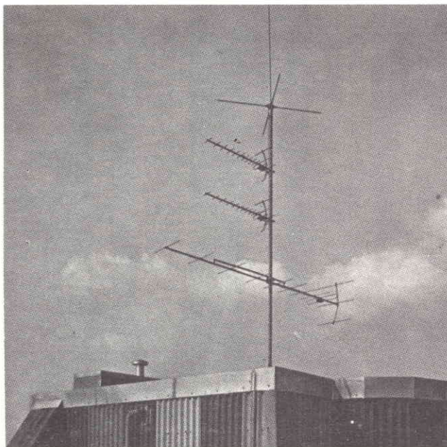
Fig. 3 - Parte visibile di un impianto d'antenna centralizzato. Su un palo sono sistemate più antenne televisive differenti. Alla sommità del palo si nota un'antenna radio.
