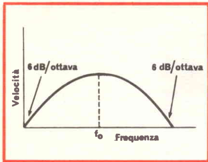
Fig. 9 - Curva di risonanza di un trasduttore a velocità costante.
