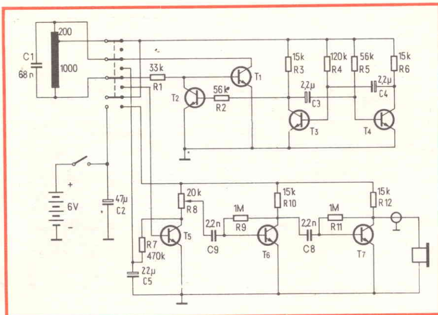
Fig. 3 - Schema elettrico del «Piep I».
