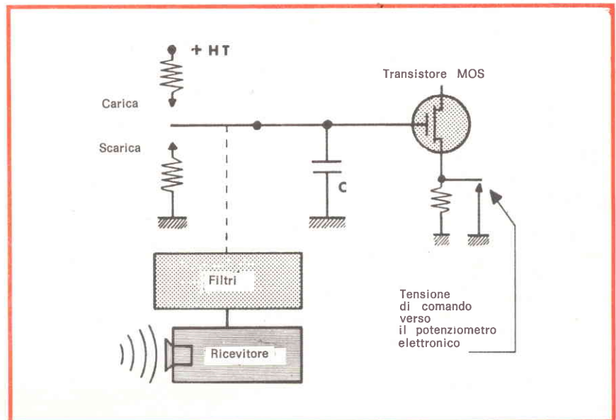
Fig. 9 - Il potenziometro di figura 8 può essere sostituito da un sistema elettronico comandato da una tensione continua. Questa tensione è fornita dal dispositivo sopra indicato. Il ricevitore comanda un invertitore (che può essere esso stesso elettronico) il quale a sua volta carica o scarica un condensatore.
