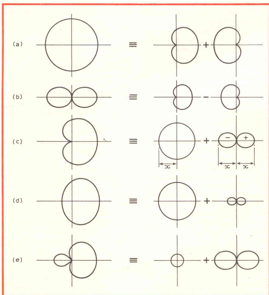
Fig. 8 - Schemi di vari diagrammi polari (a) omnidirezionale, (b) bidirezionale ad otto, (c) unidirezionale o cardiode, (d) supercardioidale ed (e) ipercardioidale.
