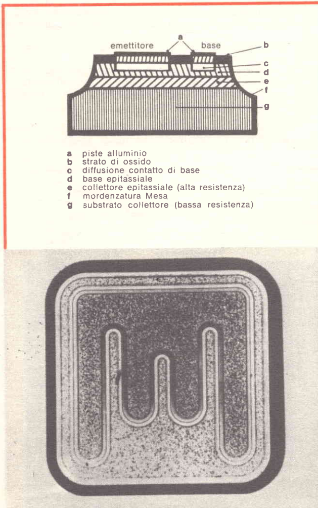
Fig. 27 - (in alto) Sezione schematica di un transistoro epitassiale; (in basso) strato epitassiale prima dell'applicazione delle piste di alluminio per i contatti rispettivamente di base e di emettitore.
