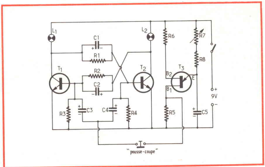
Fig. 11 - Nello schema elettrico del dispositivo elettronico si nota l'impiego di tre soli transistori, di cui due costituiscono il multivibratore (T1 e T2), e l'altro (T3) il generatore di impulsi che comanda il multivibratore attraverso il pulsante.
