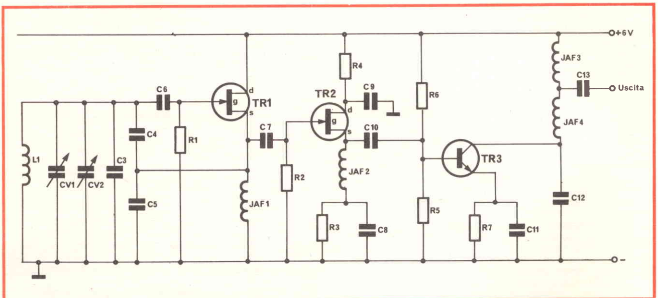
Fig. 1 - Schema elettrico del VFO a transistori FET descritto in questo articolo.
