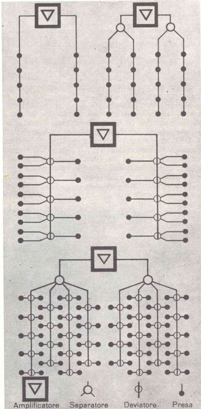
Fig. 8 - Gli schemi danno un'idea della molteplicità delle discese in cavo di reti di distribuzione. La scelta della soluzione migliore dal punto di vista tecnico ed economico è frutto di adeguate cognizioni tecniche e dell'esperienza.
