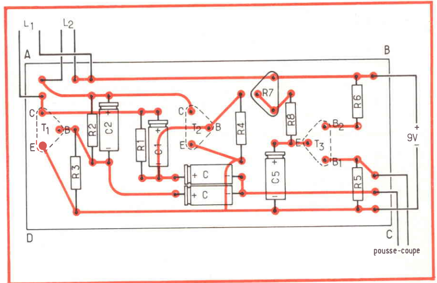
Fig. 12 - Montaggio dei componenti sul circuito stampato.
