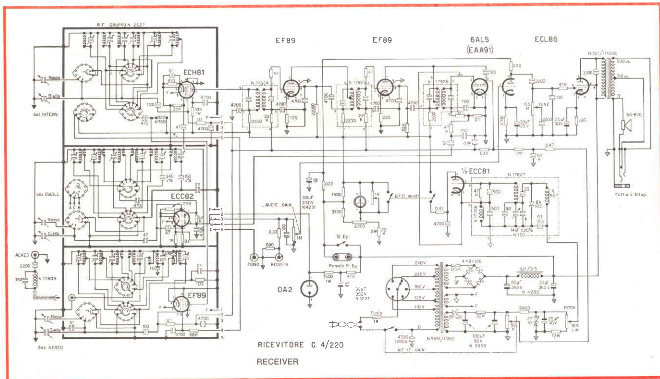
Fig. 2 - Schema elettrico di un apparecchio a valvole per onde medie e corte modello G 4/220 della Geloso, la cui tabella delle tensioni è riportata nel testo.
