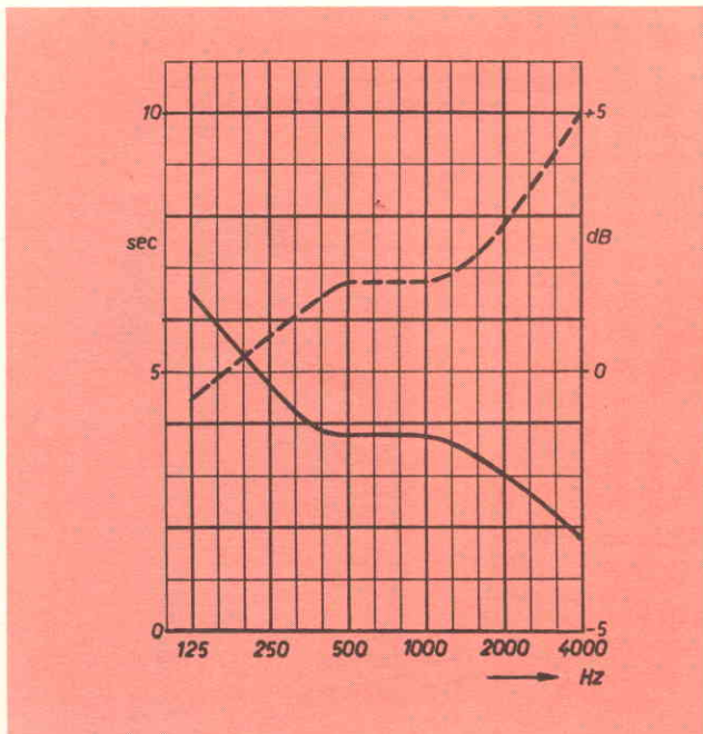
Fig. 2 - Tempo di riverberazione in sec (linea continua) e fattore di ambiente in dB (linea tratteggiata) della camera di figura 1.
