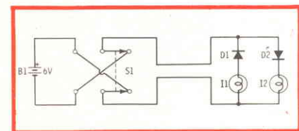
Fig. 10 - Comando a distanza di due circuiti distinti mediante l'impiego di due soli conduttori.
