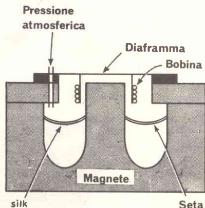
Fig. 11 - Schema costruttivo del microfono a bobina mobile.
