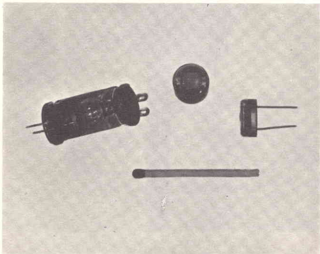
Fig. 36 - Fotoresistenza RPY33 al solfuro di cadmio con sensibilità in testa (Philips).
