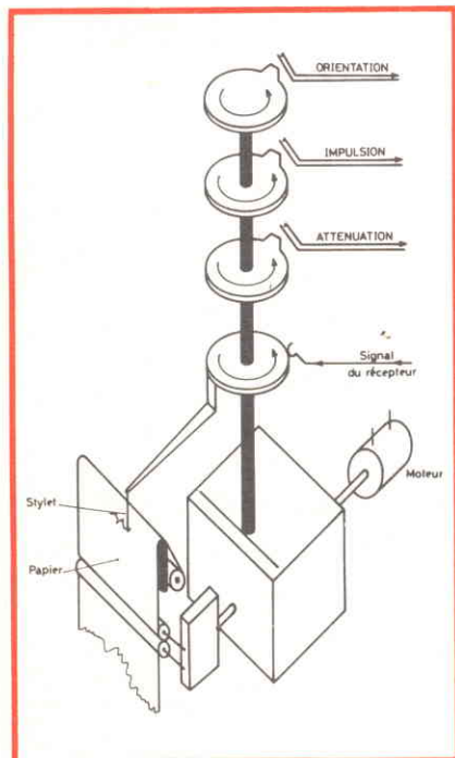
Fig. 22 - Per registrare gli impulsi riflessi forniti dall'impianto Sonar, nonché i dati relativi all'orientamento, agli impulsi ed all'attenuazione, si fa uso di un sistema di registrazione del tipo il cui principio di funzionamento viene chiarito in questa figura.
