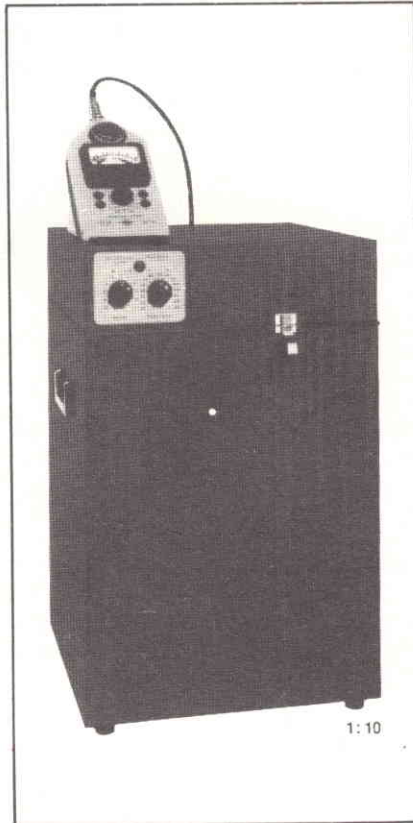
Fig. 11 - Piccola camera anecoica per la prova delle protesi auditive.
