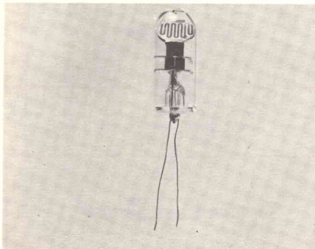
Fig. 33 - Sfruttamento dell'effetto fotoelettrico «interno» nella cellula fotoconduttrice (o fotoresistenza) al solfuro di cadmio ORP 50 (a sinistra) e all'antimoniuro di indio ORP 10 (a destra).
