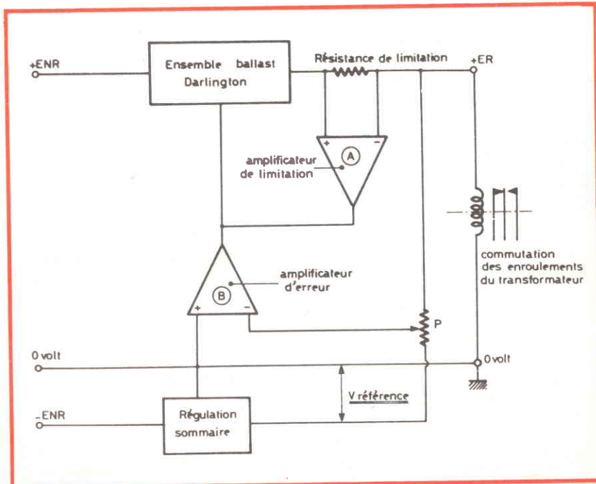
Fig. 16 - Principio schematico di funzionamento dell'alimentatore stabilizzato descritto sulla Rivista francese, in grado di fornire in uscita una tensione regolabile da 0 a 30 V.
