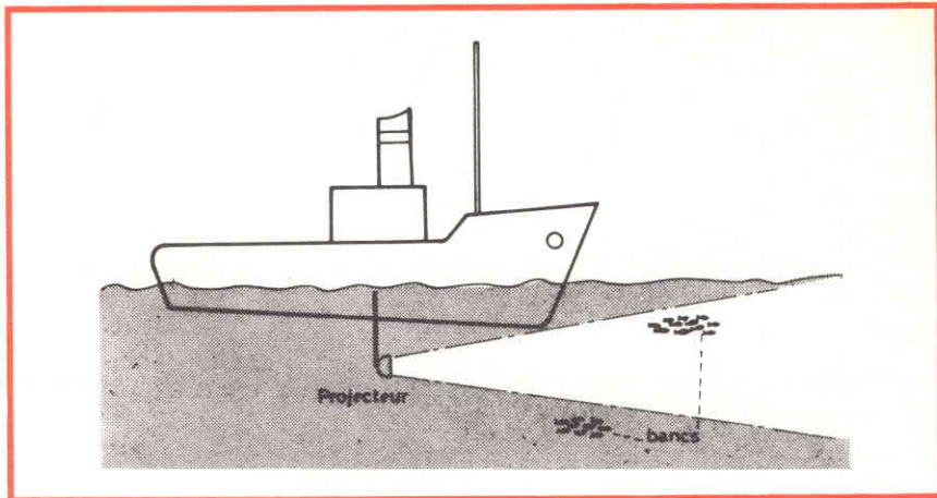
Fig. 19 - Principio di funzionamento del Sonar, basato sull'impiego di un proiettore che invia un raggio di onde ultrasoniche, che viene riflesso verso il proiettore stesso quando viene intercettato un ostacolo fisso o mobile.
