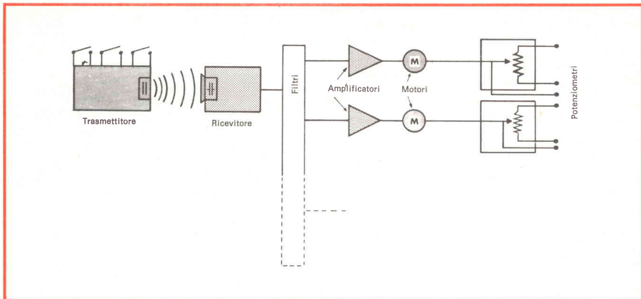
Fig. 6 - Telecomando ad ultrasuoni in cui ogni motore è solidale con un potenziometro che da esso viene trascinato. Il motore eccitato dal ricevitore sostituisce il comando manuale.
