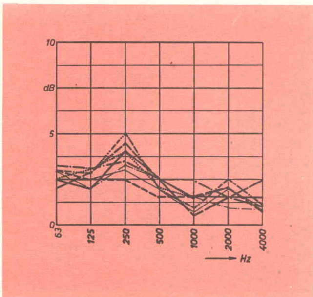
Fig. 9 - Scarto quadratico medio relativo alle distribuzioni statistiche in base alle quali è stato calcolato il livello di potenza sonora riportata in fig. 8.
