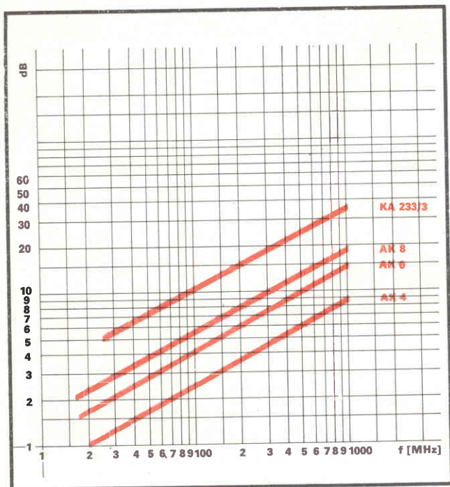
Fig. 10 - Diagrammi di attenuazione nel cavo di energia ad alta frequenza in funzione della frequenza in alcuni tipi di cavi Eltronik.
