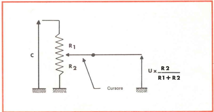
Fig. 8 - Un potenziometro può essere scomposto in due resistori variabili la cui somma di valori è costante. La tensione ai capi del cursore viene variata dalla posizione di quest'ultimo.
