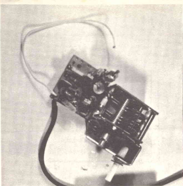
Fig. 5 - Prototipo del VFO a realizzazione ultimata.
