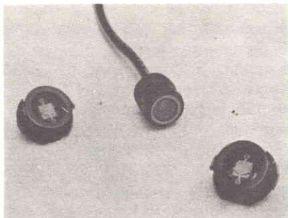
Fig. 2 - Due tipi di trasduttori utilizzati con gli ultrasuoni. Al centro, un microfono (o altoparlante) elettrostatico utilizzato dalla Grundig. Ai due lati trasduttori piezo-elettrici. Nei due casi, una griglia metallica lascia passare gli ultrasuoni e protegge le parti attive relativamente fragili.
