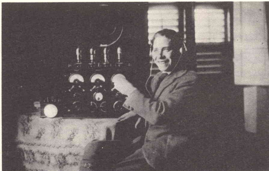
Fig. 3 - 8-GF vicino al suo ricevitore con quattro cipolloni e dieci comandi, oltre al celebre altoparlante a tromba.
