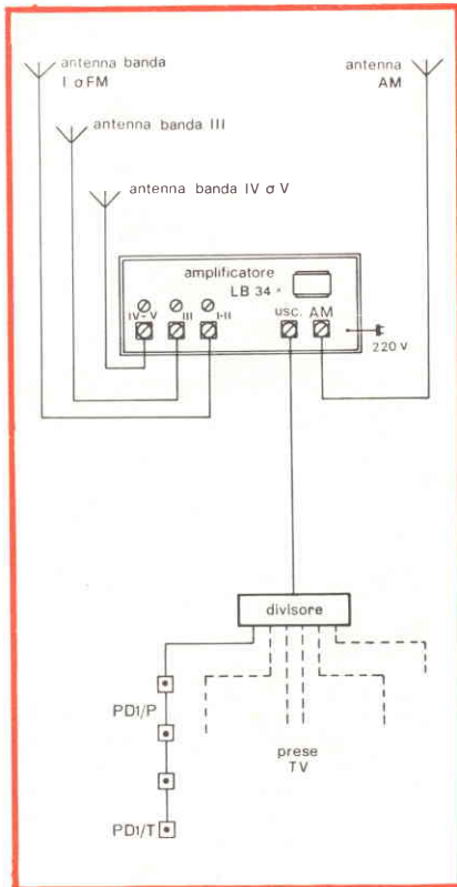
Fig. 5 - Disposizione schematica dell'impianto di cui alla figura 4. Le sigle dei divisori e delle prese si riferiscono al codice della Prestel. Tali componenti sono reperibili presso la GBC Italiana.
