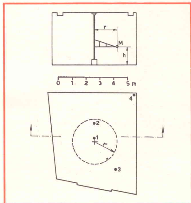
Fig. 3 - Schema del dispositivo rotante per il rilievo del livello di pressione sonora medio L_{pm} .
