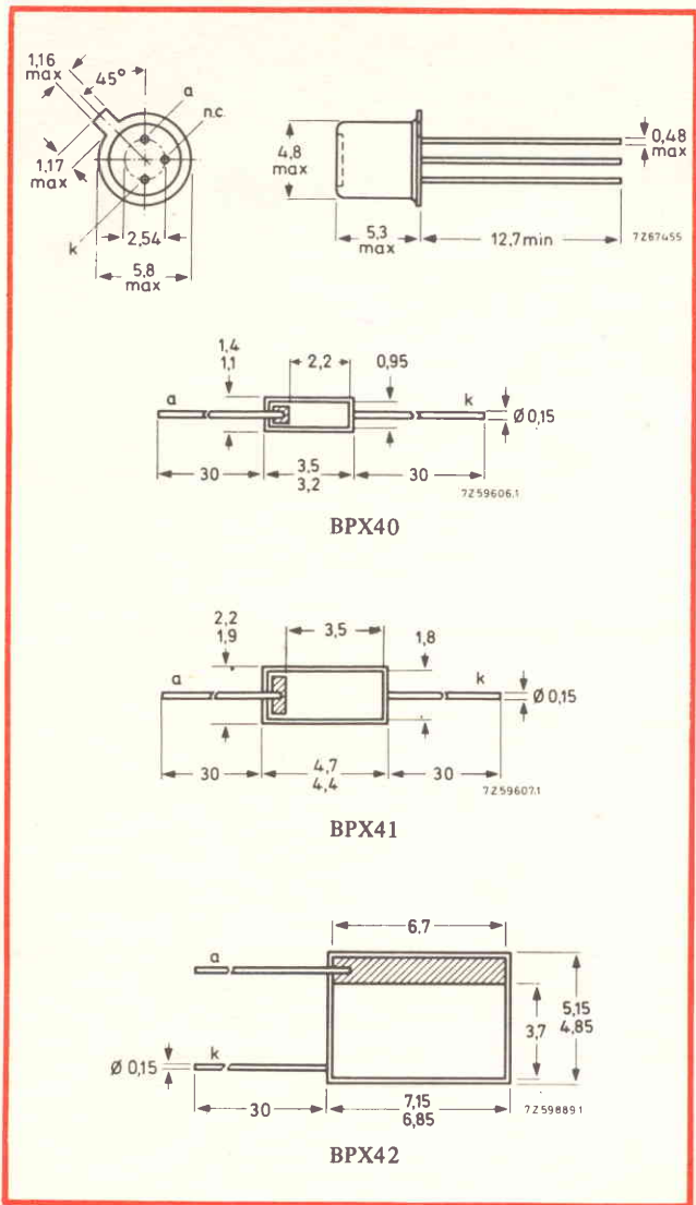
Fig. 32 - Contenitori di alcuni tipi di fotodiodi di produzione europea.
