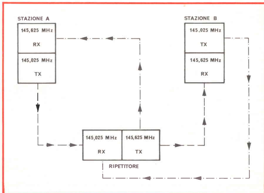
Fig. 1 - Schema di principio relativo al funzionamento dei ponti radio, norme IARU, per radioamatori, con differenza di frequenza RX - TX di 60 kHz.
