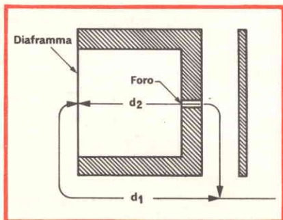
Fig. 6 - Microfono a spostamento di fase.
