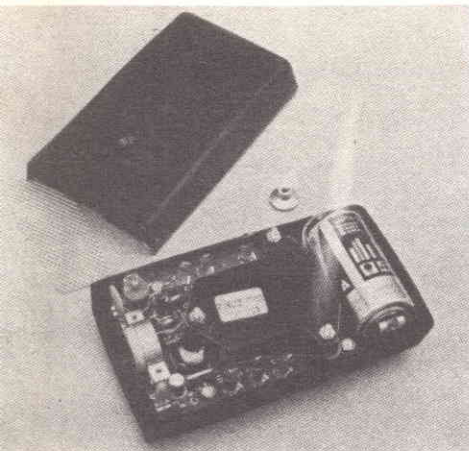
Fig. 11 - Il trasmettitore Grundig impiega un numero limitato di componenti. L'alimentazione è ottenuta da una normale pila da 1,5 V. Al centro si nota la piastrina degli interruttori che inserisce nel circuito i condensatori che servono per determinare la frequenza di emissione.
