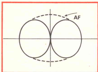
Fig. 5 - Schema polare di un microfono a gradiente di pressione.
