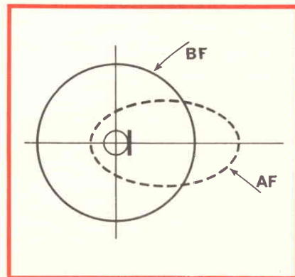
Fig. 2 - Risposta di un microfono a pressione.
