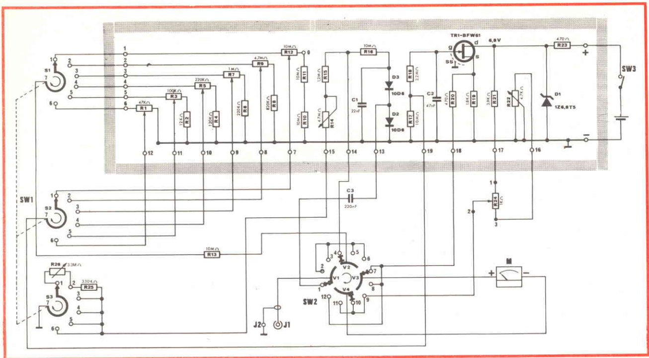
Fig. 8 - Schema elettrico del voltmetro elettronico UK 475/C della AMTRON, reperibile in kit presso la GBC Italiana.
