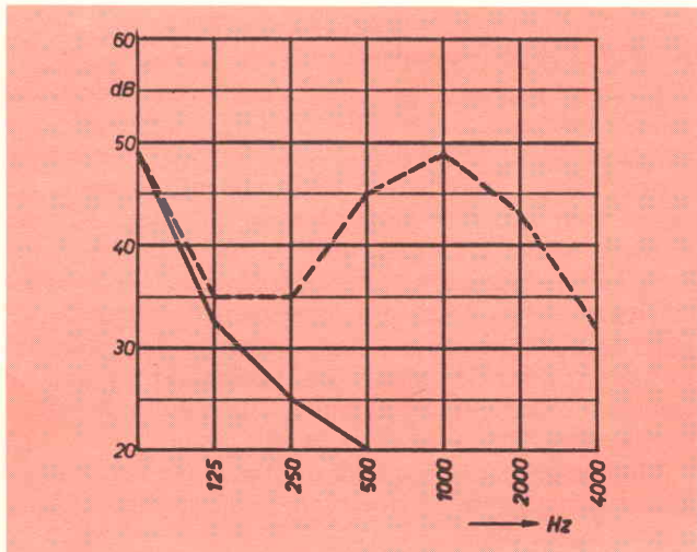
Fig. 4 - Livello del rumore di fondo dell'ambiente di misura con il sistema rotante fermo (linea continua) e in funzione (linea tratteggiata).
