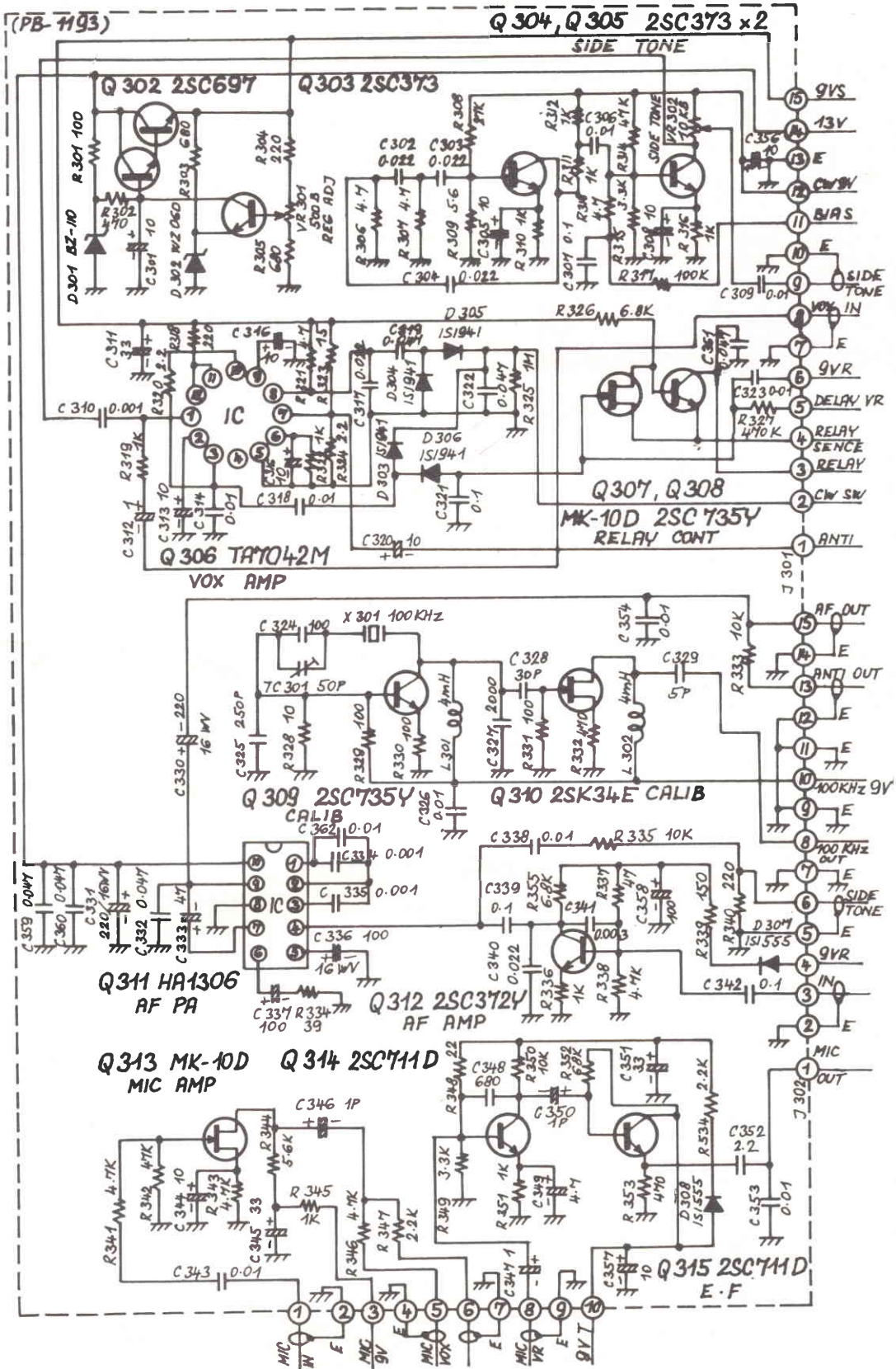
Fig. 4 - Schema elettrico della sezione BF audio, Calibratore a 100 kHz, Preamplificatore microfonico e circuiti Vox, Antitrip e Sidetone.
