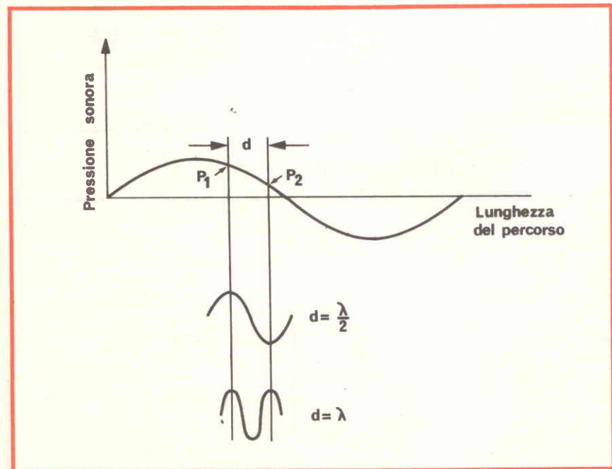
Fig. 4 - Relazione esistente fra pressione sonora e lunghezza del percorso nei microfoni a gradiente di pressione.
