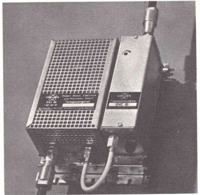
Fig. 9 - Amplificatore Elektronik della Robert Bosch per grandi impianti centralizzati.
