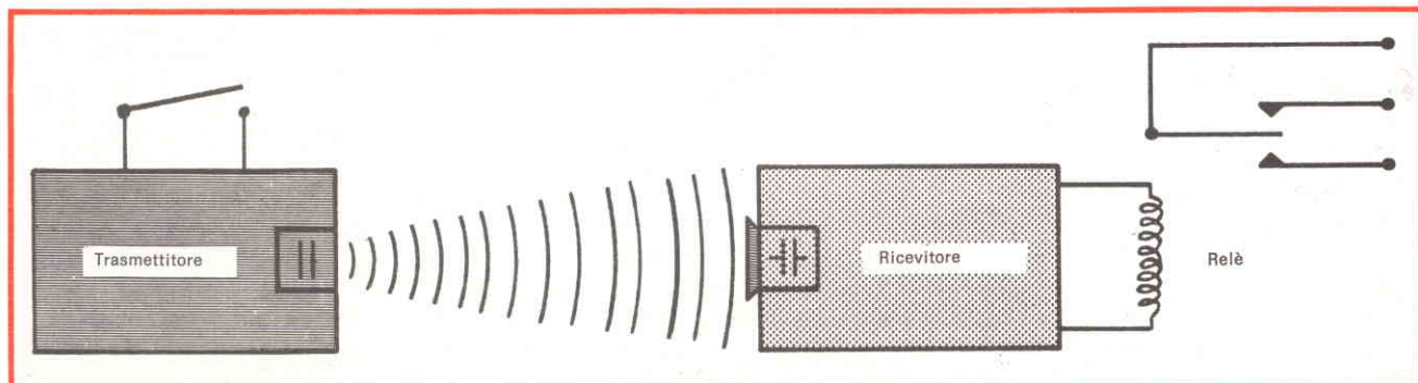
Fig. 3 - Il più semplice sistema concepibile: un trasmettitore con un tasto di comando e un ricevitore che aziona i contatti di un relè.
