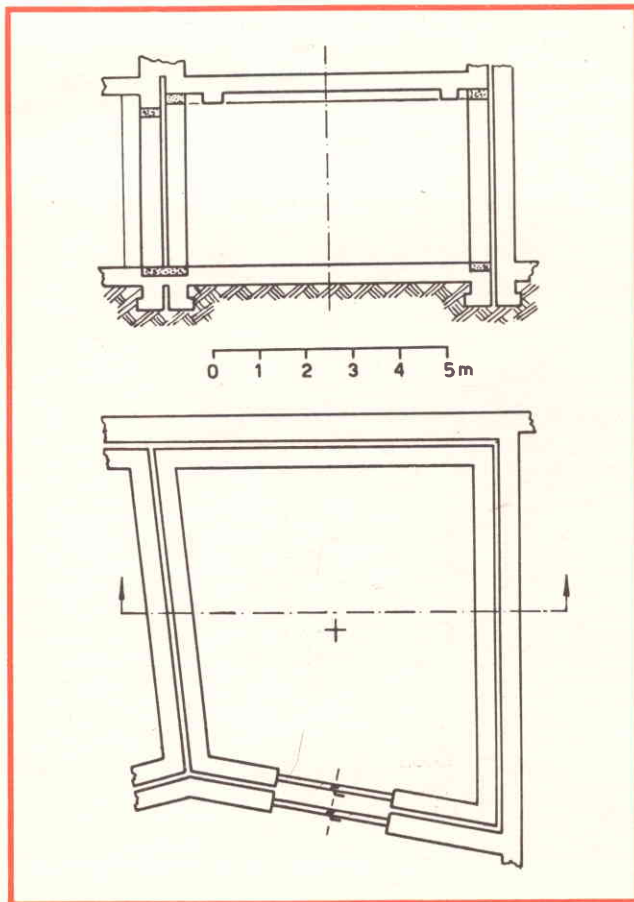
Fig. 1 - Sezione e pianta della camera riverberante di misura.
