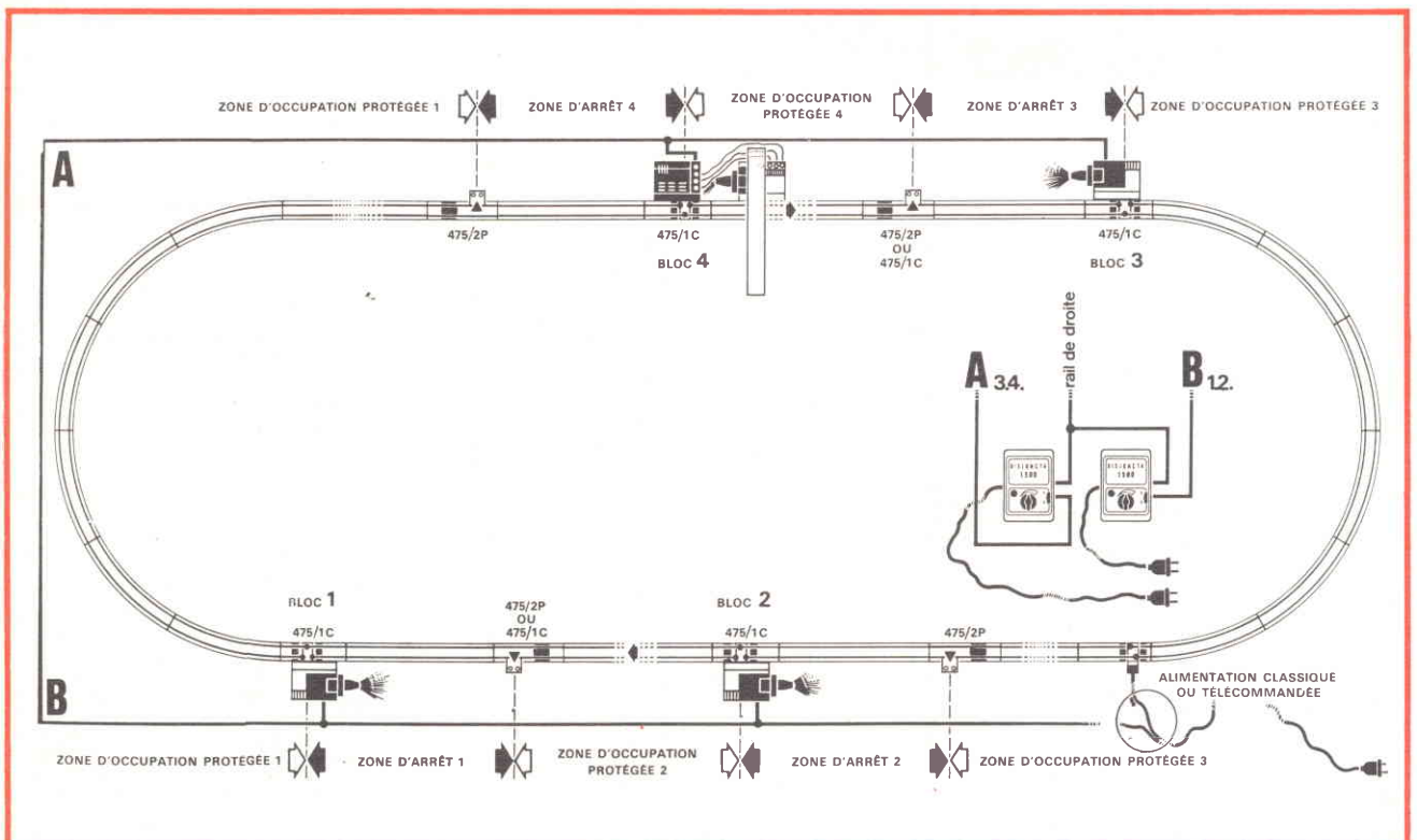
Fig. 3 - Sistema integrale di bloccaggio, facente uso di sistemi di segnalazione del tipo visibile all'interno del circuito ferroviario, verso il lato destro.
