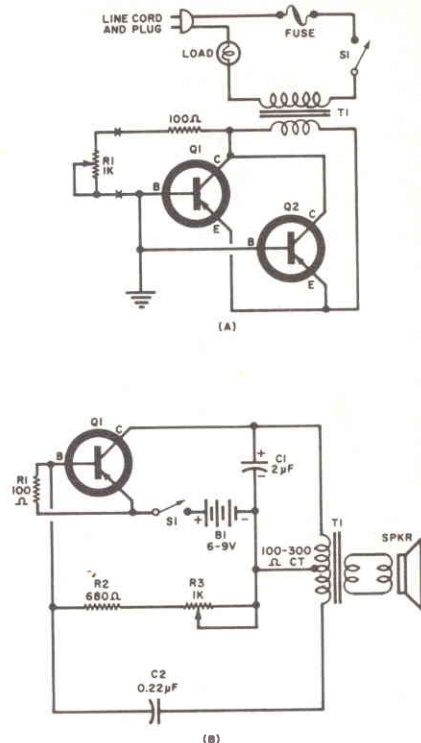
Fig. 7 - Esempio di semplice circuito elettronico di potenza per il comando di piccoli motori elettrici (A), e semplice circuito per la produzione di una nota a frequenza costante, dai molteplici impieghi (B).
