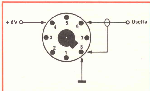
Fig. 4 - Presa VFO EXT del ricetrasmittitore Sommerkamp FT-277.
