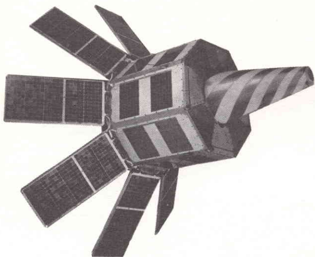
Fig. 39 - Batteria di celle solari al silicio BPX33 (Philips) per impieghi spaziali.
