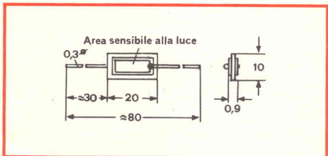
Fig. 37 - Dimensioni della cella solare al silicio BPY45 (Siemens).
