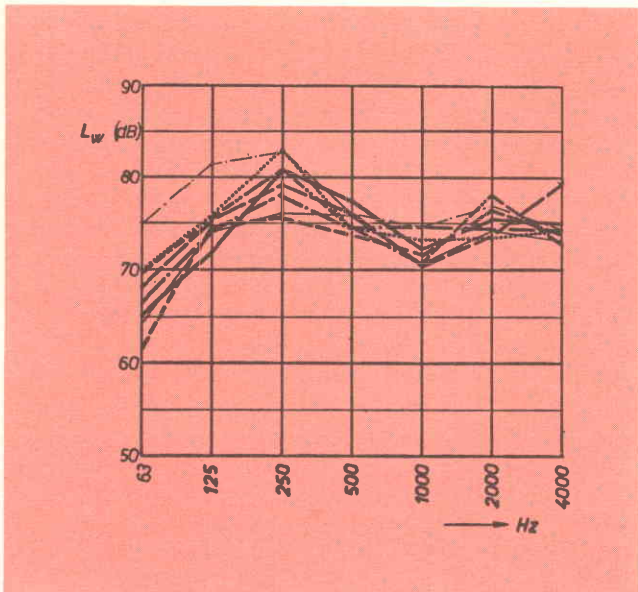
Fig. 8 - Livello di potenza sonora di un aspirapolvere, dedotto da diverse misure in camera riverberante. (La linea a tratto e punto sottile corrisponde ad una misura con sorgente al centro della camera).
