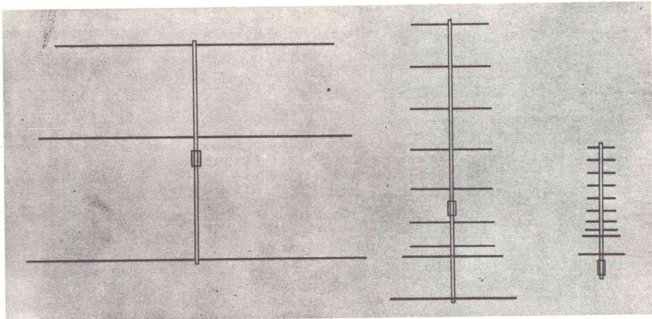
Fig. 4 - Antenne televisive per la ricezione di differenti lunghezze d'onda. Da sinistra a destra: TV I, TV III, TV V.
