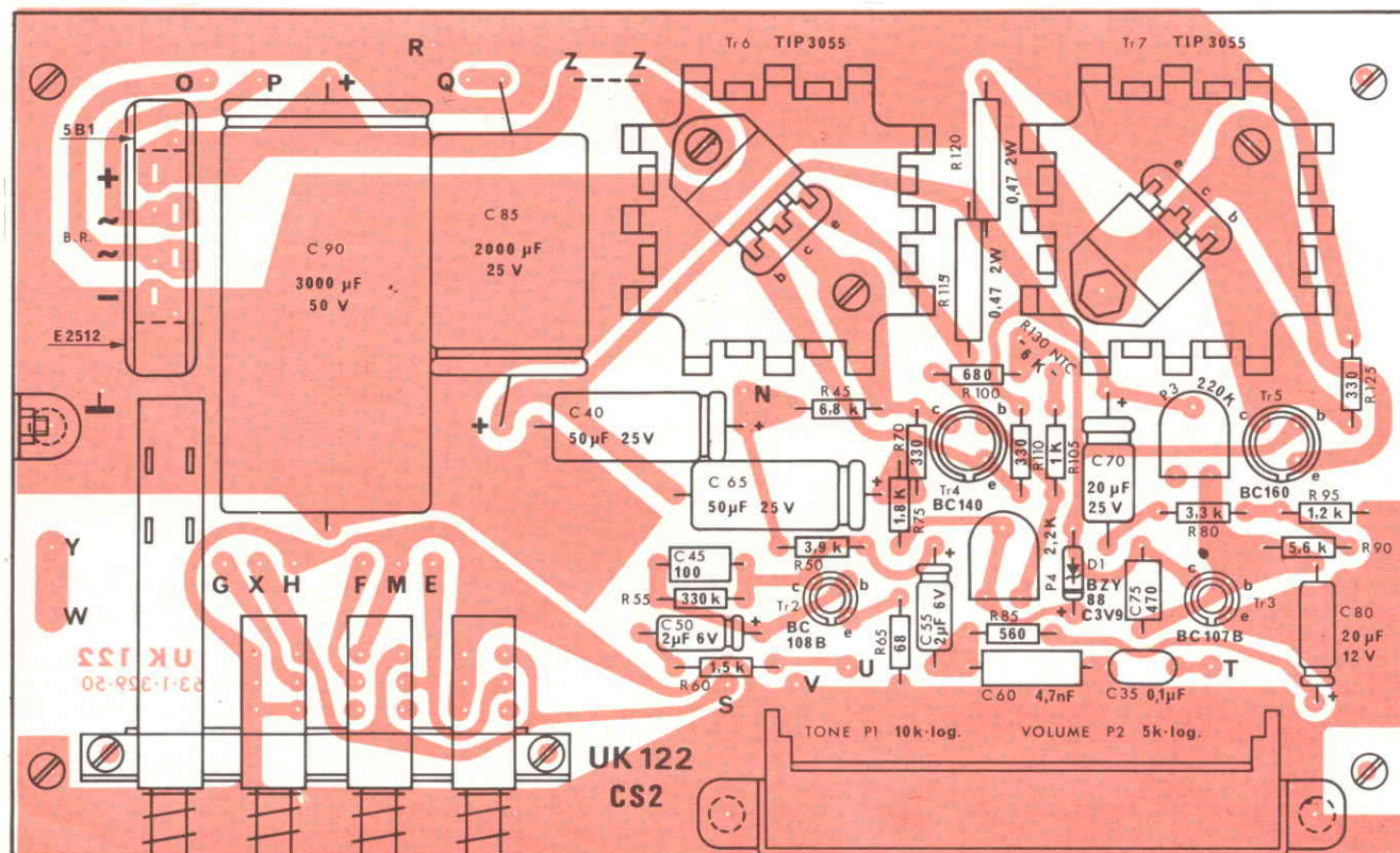
Fig. 3 - Disposizione dei componenti sulla basetta a circuito stampato C.S.2.
