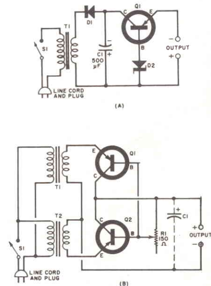
Fig. 8 - In alto (A) è illustrato lo schema elettrico di un piccolo alimentatore regolato, facente uso come elementi di regolazione di un solo transistor, e di un diodo zener. In basso (B) è invece illustrato lo schema di un altro tipo di alimentatore regolato, che può essere usato sia per la ricarica di batterie, sia per alimentare circuiti elettronici sperimentali.
