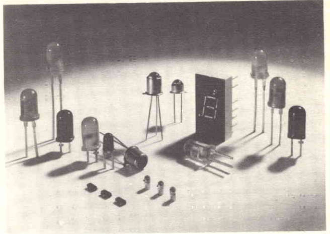
Fig. 28 - (in basso a destra) fotodiodi e fototransistori; LED (Light Emitting Diode) singoli e per display (Philips).
