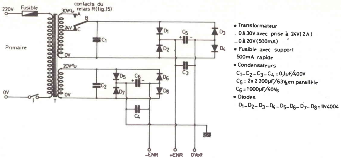
Fig. 17 - La prima parte dell'alimentatore consiste in un trasformatore provvisto di due secondari seguiti da una cellula di rettificazione a ponte e da un sistema di filtraggio, in modo da ottenere in totale due uscite, di cui una positiva ed una negativa rispetto a massa.
