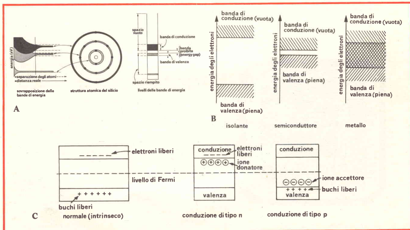
Fig. 26 - a) bande di energia nel silicio; b) bande di energia in un materiale isolante, semiconduttore e conduttore; c) effetto del drogaggio sulle bande di energia di un materiale semiconduttore.
