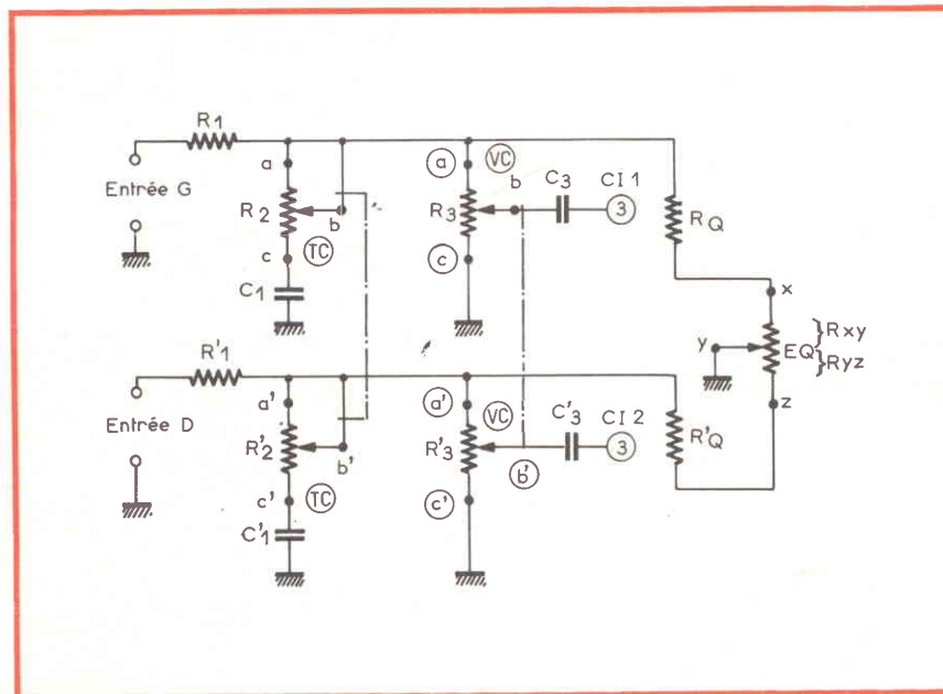
Fig. 10 - Metodo di allestimento del doppio circuito di ingresso per i due canali destro e sinistro, che può comportare comandi unici ed abbinati tra loro, oppure comandi unici ma indipendenti, muniti cioè di perni di comando coassiali. A destra è visibile il potenziometro per il controllo del bilanciamento, che può essere soppresso se i due controlli di volume agiscono separatamente.
