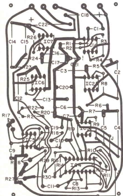
Fig. 6 - Disposizione dei componenti sulla basetta a circuiti stampati.
