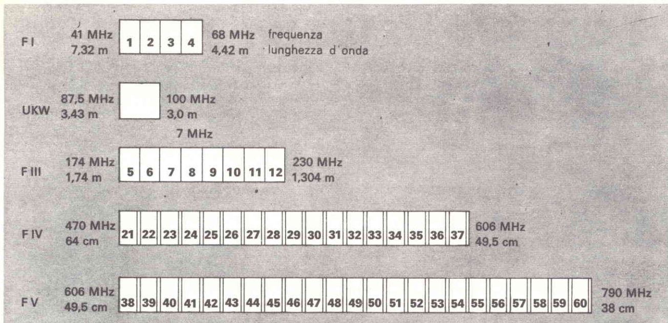
Fig. 2 - Bande di frequenza, canali e lunghezza d'onda relative alle trasmissioni televisive.
