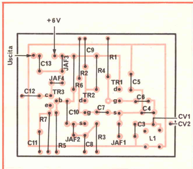
Fig. 3 - Disposizione dei componenti sul circuito stampato di fig. 2.
