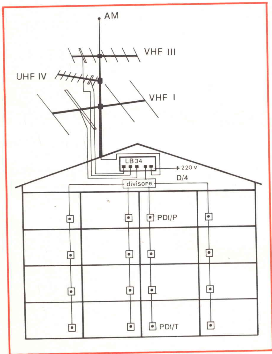
Fig. 4 - Impianto di amplificazione per programmi televisivi. E' possibile la ricezione di due canali VHF e uno UHF con centralino a larga banda con entrata per antenna AM.
