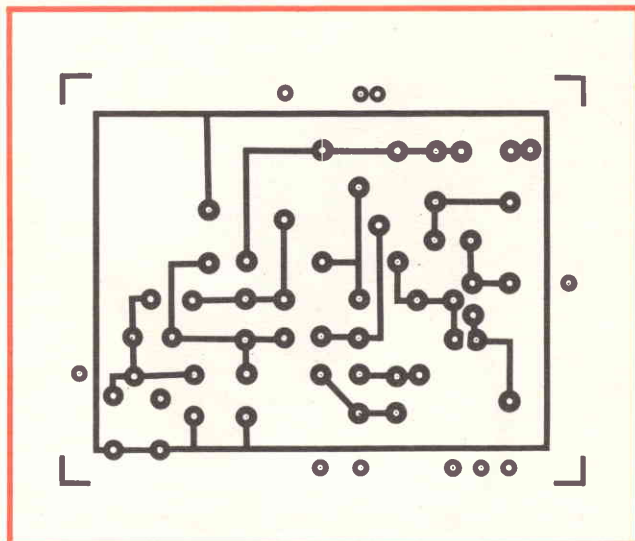
Fig. 2 - Circuito stampato in grandezza naturale visto dal lato rame.
