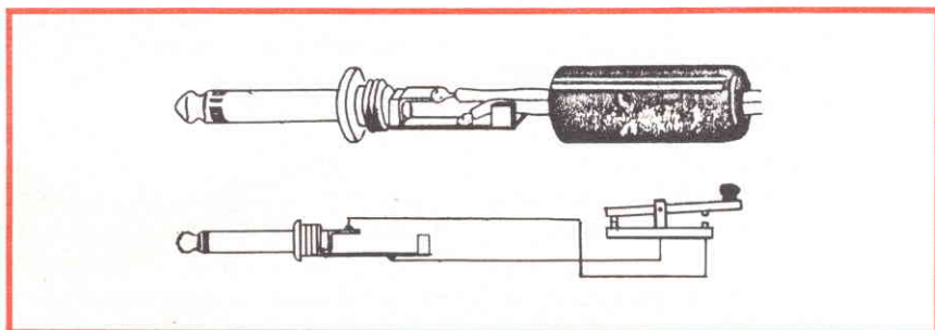
Fig. 1 - Collegamenti da effettuare alla spina del tasto telegrafico.
