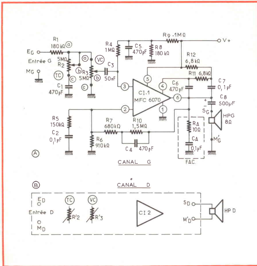
Fig. 9 - Circuito elettrico completo di una delle sezioni che costituiscono il modulo stereofonico. In basso è riprodotto simbolicamente l'altro canale costituito da una unità del tutto identica.
