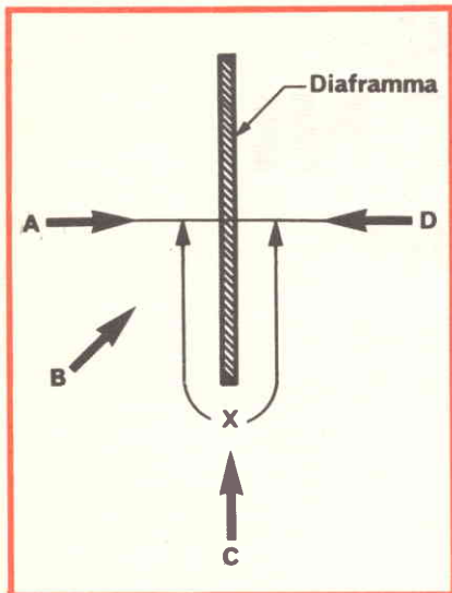
Fig. 3 - Microfono a gradiente di pressione.
