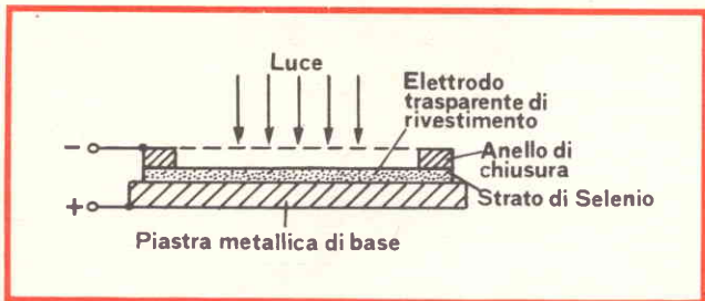
Fig. 35 - Struttura schematica di una fotoresistenza.
