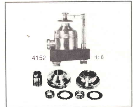
Fig. 13 - Orecchio artificiale B & K, per misure su audiometri, cuffie, e ricevitori per deboli di udito.
