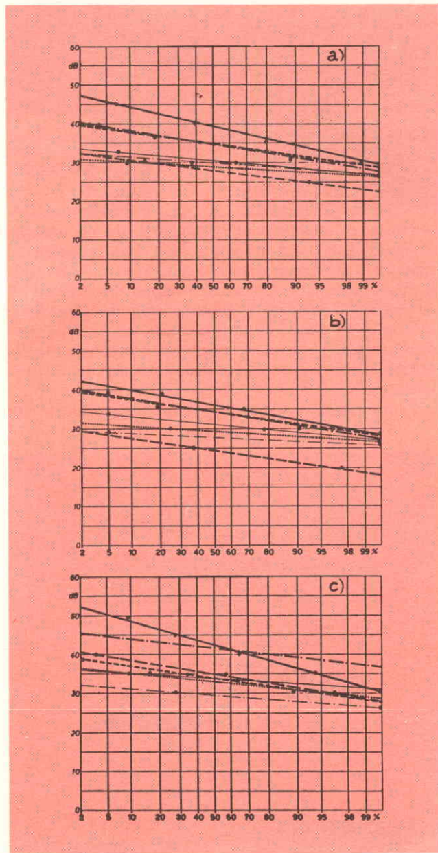
Fig. 7 - Distribuzione statistica dei livelli relativi di pressione sonora per un aspirapolvere posto rispettivamente nei punti 4 (a), 3 (b) e 1 (c). Posizione del microfono: h = 1,3 m, di figura 2.
