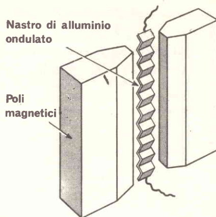
Fig. 12 - Principi costruttivi del microfono a nastro.
