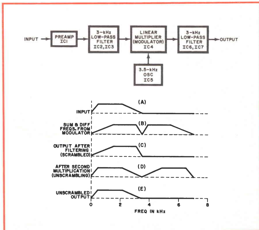
Fig. 5-A - Schema a blocchi illustrante il principio di funzionamento del dispositivo di codificazione delle comunicazioni telefoniche, e l'andamento dei cicli di inversione delle frequenze, espressi graficamente.
