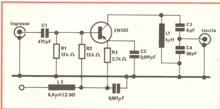
Fig. 1 - Schema elettrico del preamplificatore per la gamma VHF ed eventualmente gamme onde corte.
