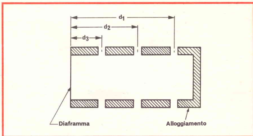
Fig. 7 - Microfono a spostamento di fase con varie aperture per ottenere una risposta più ampia.
