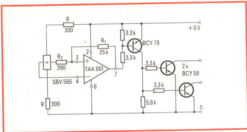
Fig. 2 - Schema elettrico relativo ad un tasto magnetico con SBV 566 della Siemens per tastiere.
