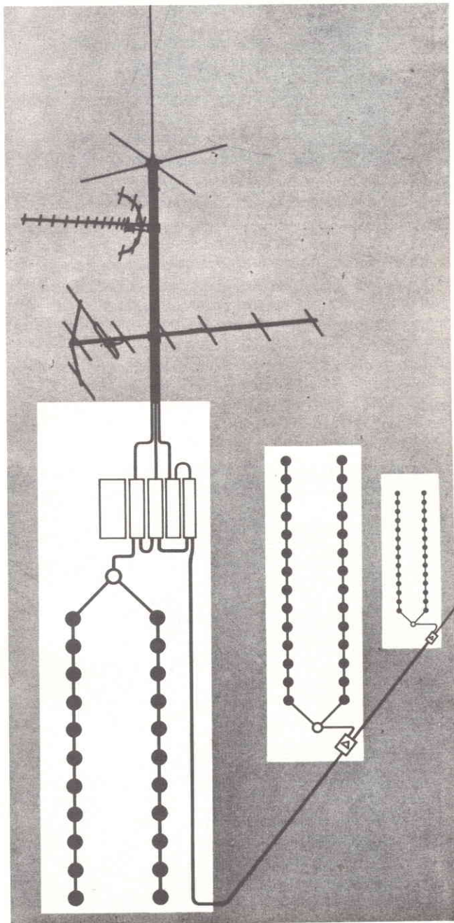
Fig. 1 - Tipica struttura di un impianto d'antenna centralizzato.
