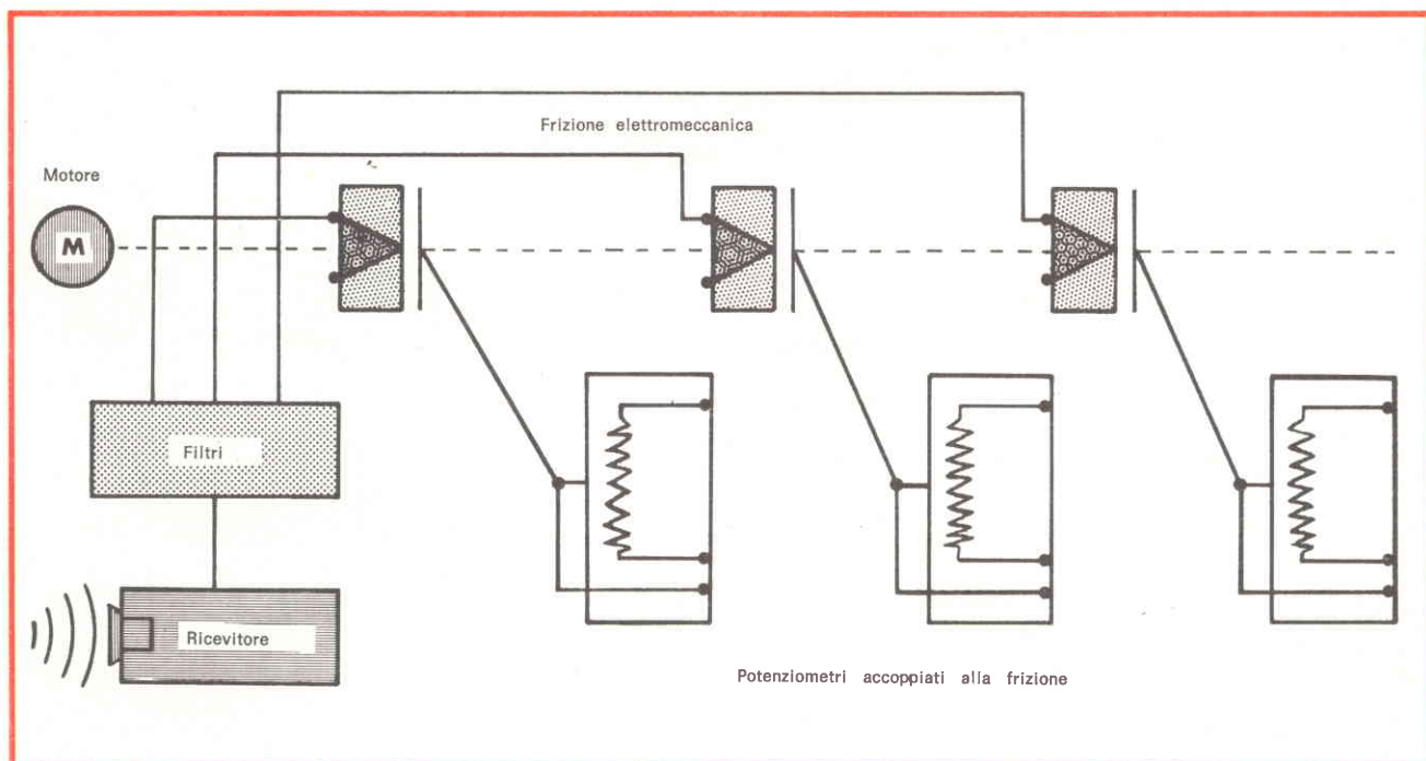
Fig. 7 - Altro principio di telecomando utilizzato in televisione e in Hi-Fi. Un solo motore trascina un'asse su cui sono montati più frizioni elettromeccaniche. Ogni frizione è comandata da una frequenza e agisce su un potenziometro.
