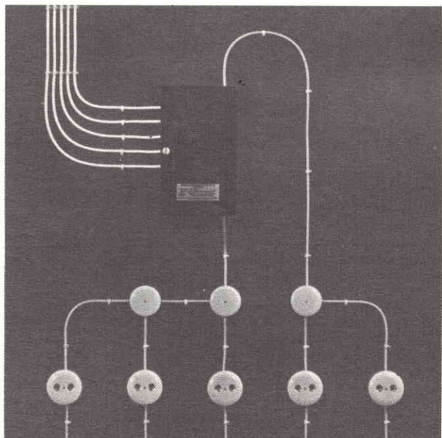
Fig. 6 - Impianto TGA1 per la ricezione radio e per quattro programmi televisivi.
